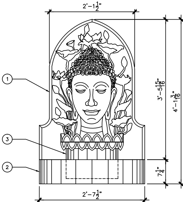
2 ELEVATION SCALE: 3/4"=1'
