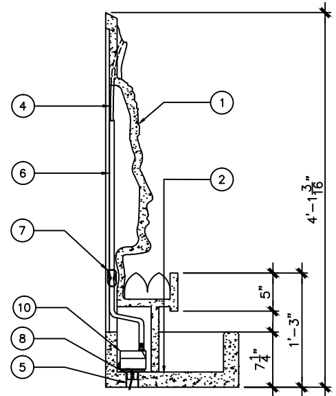
4 SECTION SCALE: 3/4"=1'
