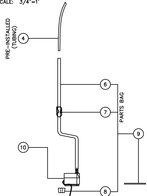
5 PIPE ASSEMBLY SCALE: 1"=1'
